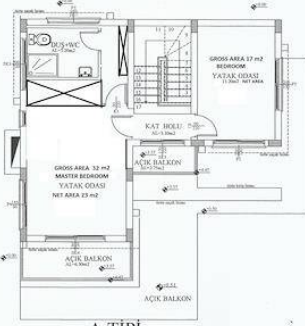
A TİPİ I. KAT PLANI ÖLÇEK 1/100 (BRÜT ALAN=58.00 m 2 )
