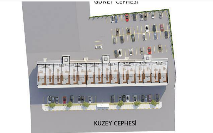
VAZİYET PLANI
